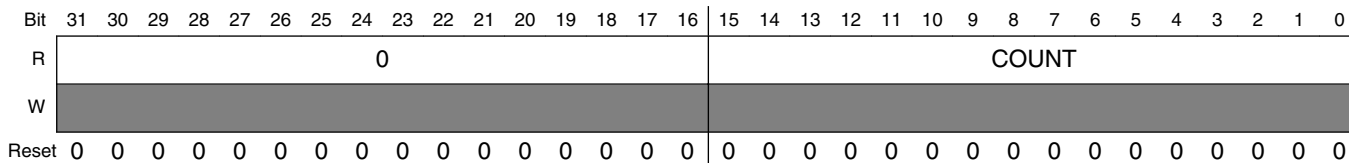
ENETx_RMON_R_BC_PKT field descriptions
