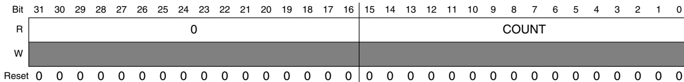
ENETx_RMON_R_MC_PKT field descriptions
